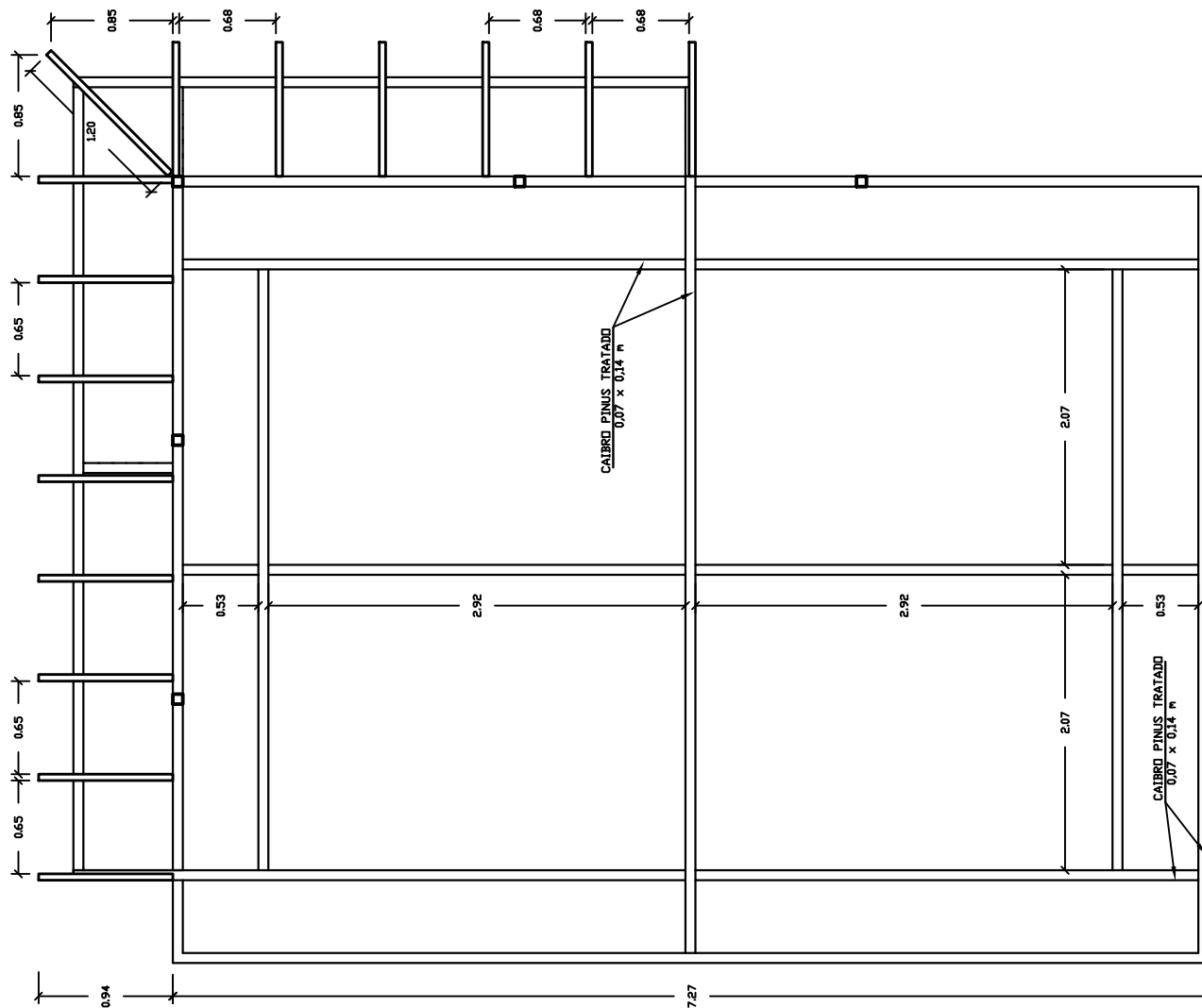
Madeiramento Cobertura Esc. 1:50
