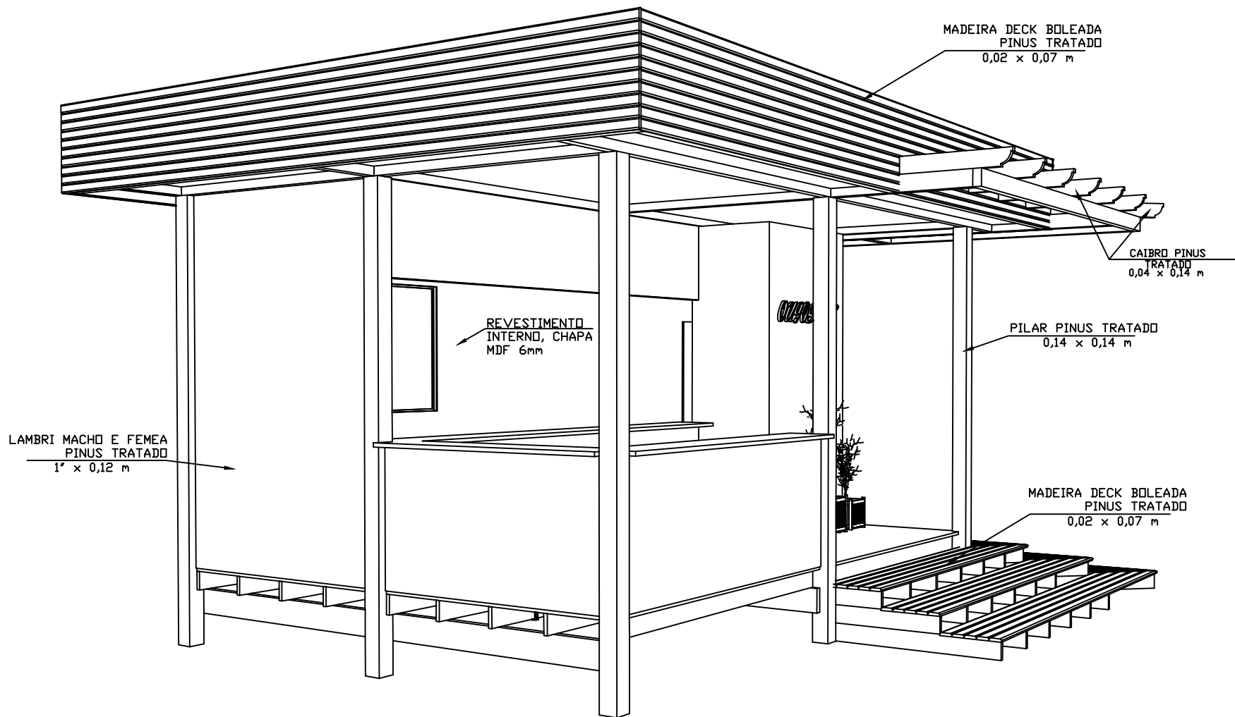
Vista isométrica Esc. 1:50
